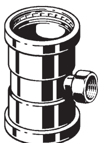
Raccordo a T Profipress XL, con SC-Contur, Modello 2417.2XL
