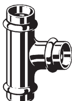
Raccordo a T Profipress G con SC-Contur, Modello 2618
