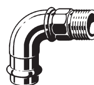
Curva a 90° Profipress G con SC-Contur, Modello 2614
