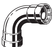
Curva a 90° Megapress con SC-Contur, Modello 4216
