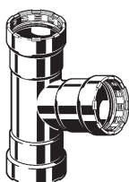
Raccordo a T Megapress S con SC-Contur, Modello 4318
