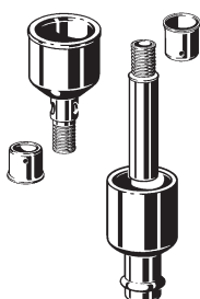
Set di allacciamento Smart-loop, Modello 2276.1
