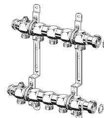
Collettore, Modello 1078
